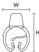
WICA-AC (Seitenansicht)
