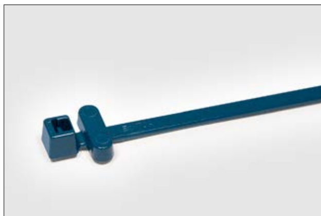
MCTRFID – detektierbare Kabelbinder mit Metallanteilen und RFID-Transponder.
